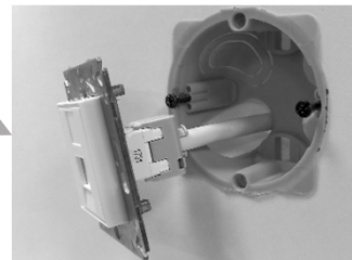
Démontez le connecteur RJ45 et ôtez la boîte d'encastrement. Réservez le câble d'origine.
