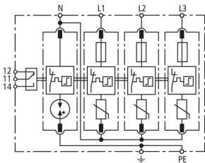
Schéma de principe du circuit DG M TT 5 CI 275 NL FM
