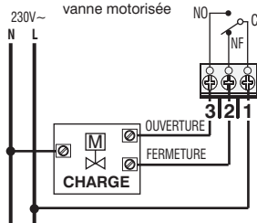
Raccordement à une vanne motorisée
